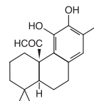
Carnosic Acid
